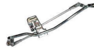
8813 DUCATO III CAM SİLECEK 1363338080 MEKANİZMASI
