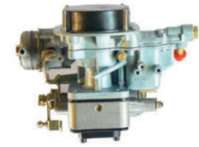
4412 1600 KARBÜRATÖR KOMPLE 85004390
